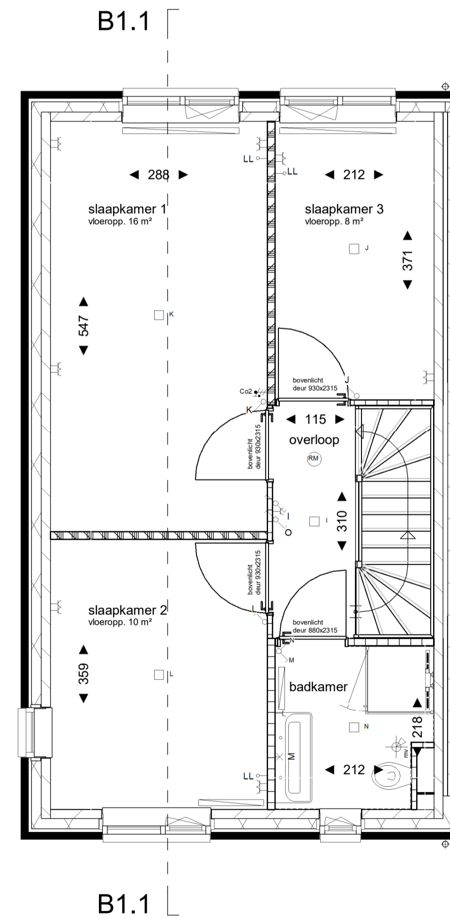
bnr: 27, 48* en 55 type Csp Eerste verdieping 1:50
