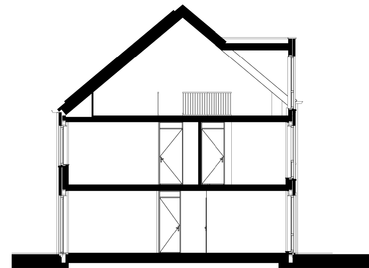
bnr: 27, 48* en 55 type Csp Doorsnede B1.1 1:100
