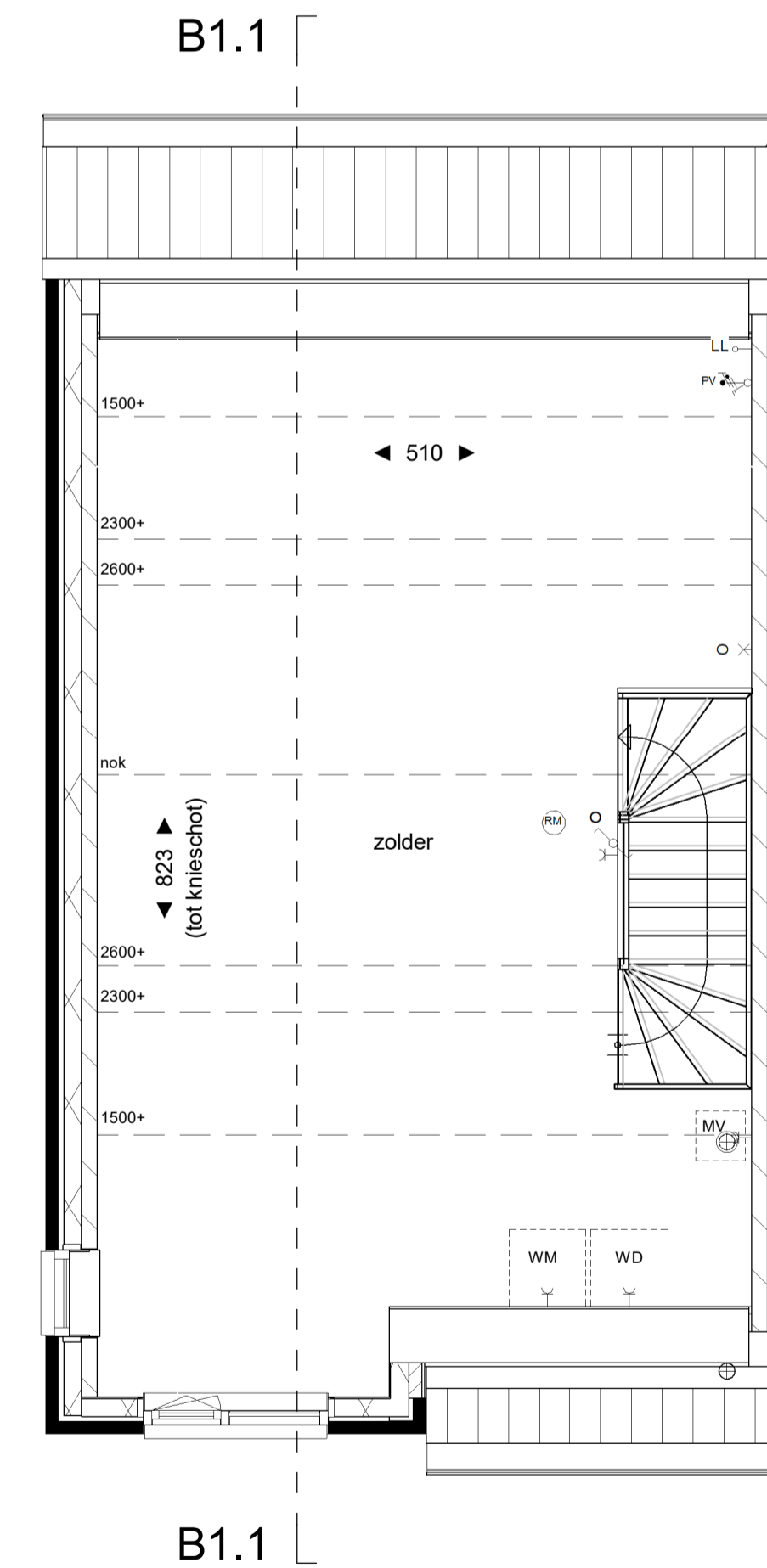
bnr: 27, 48* en 55 type Csp Tweede verdieping 1:50
