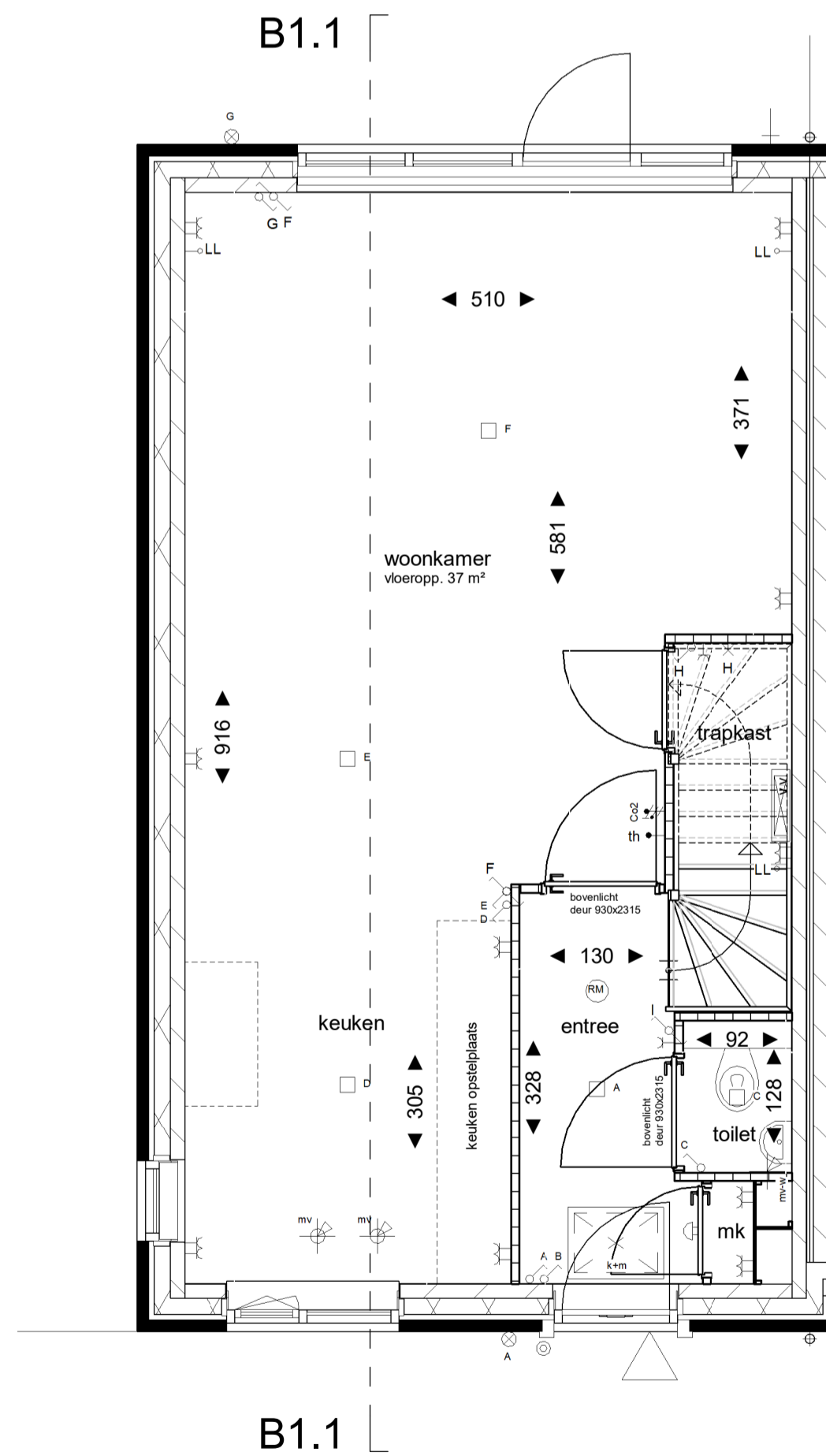
bnr: 27, 48* en 55 type Csp Begane grond 1:50
