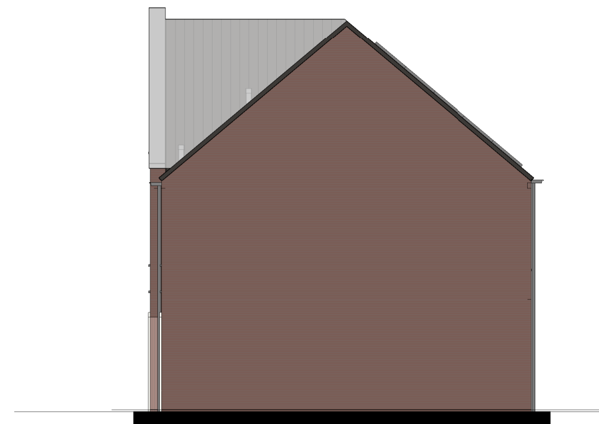
bnr: 22, 46 en 51 type C1sp Rechter zijgevel 1:100
