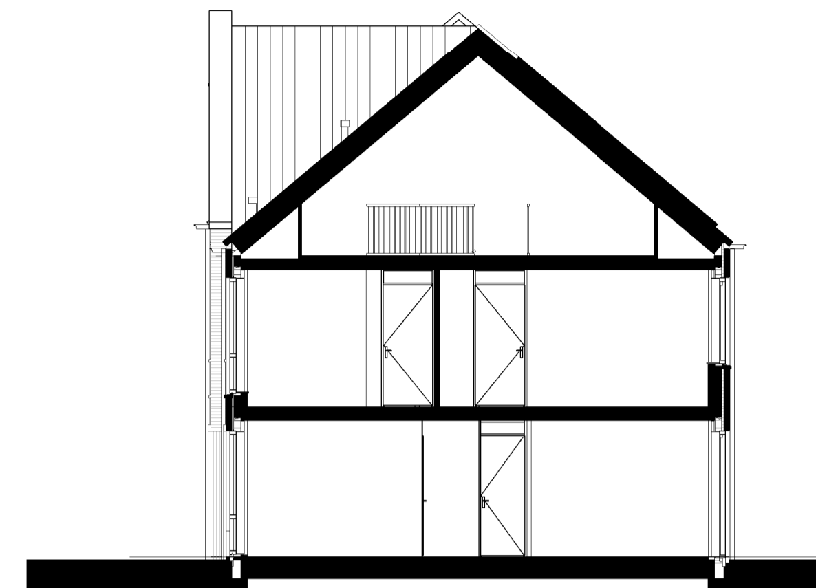
bnr: 22, 46 en 51 type C1sp Doorsnede B1.5 1:100
