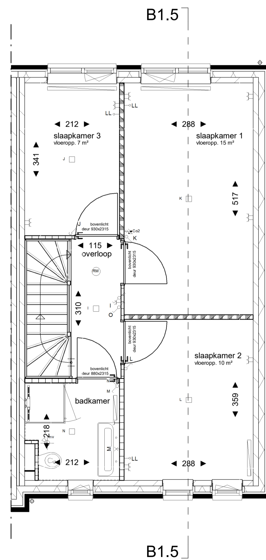
bnr: 22, 46 en 51 type C1sp Eerste verdieping 1:50
